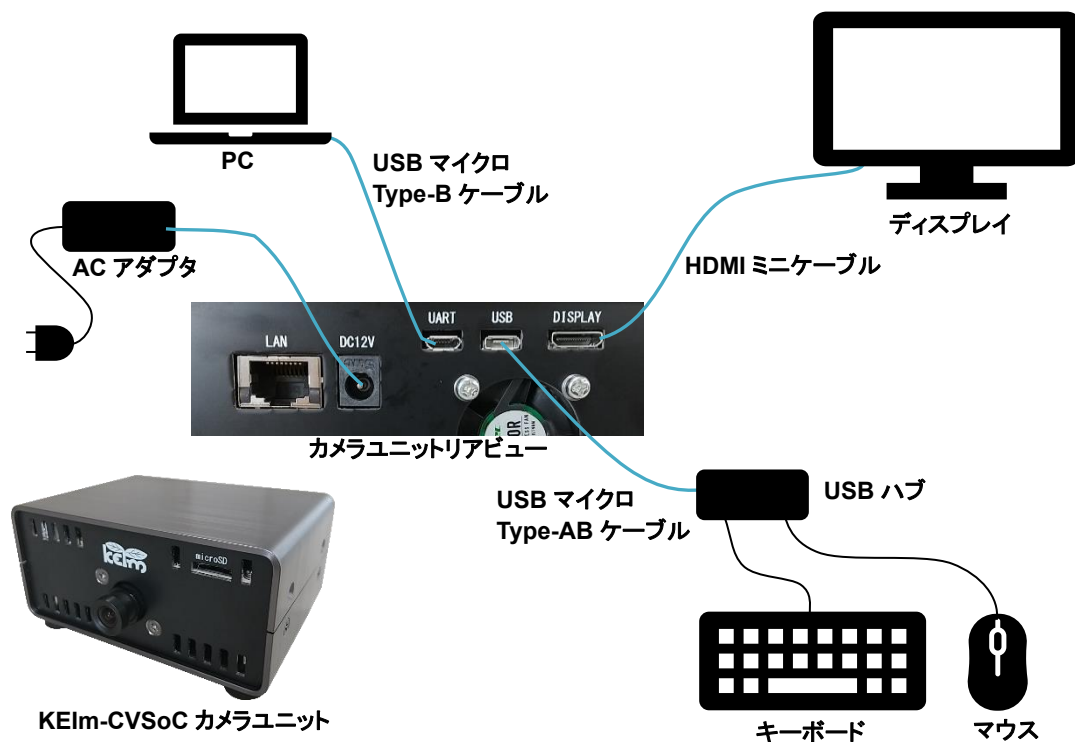
図 3-1 接続構成図
