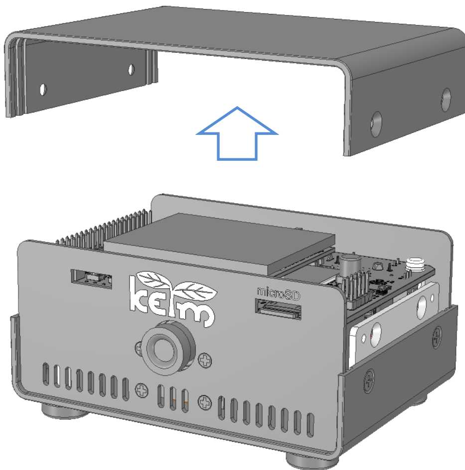
図 2-2 上蓋の取り外し
