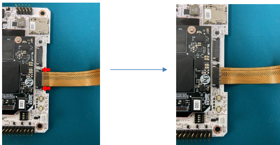
図 4-2 FPC の取り付け(IO ボード)
