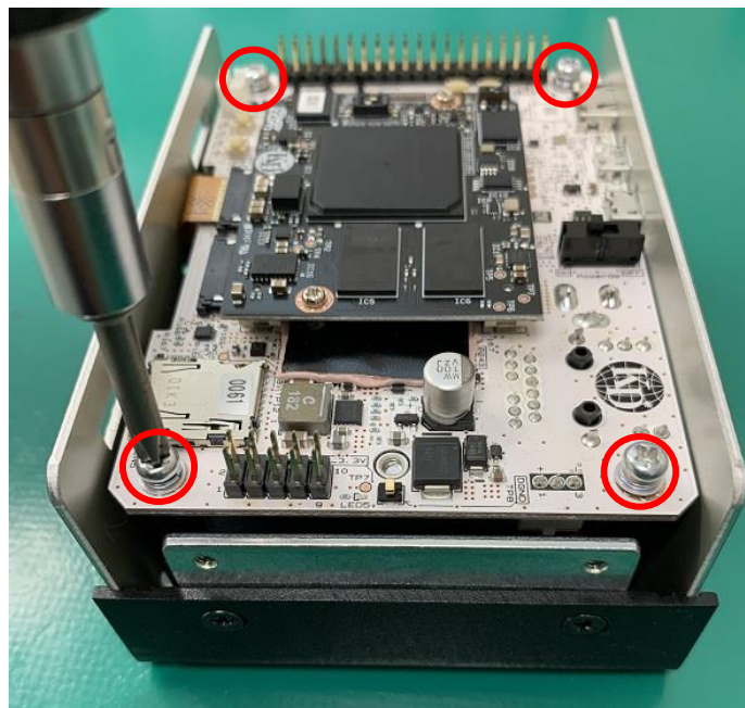
図 3-3 基板のネジ留め
