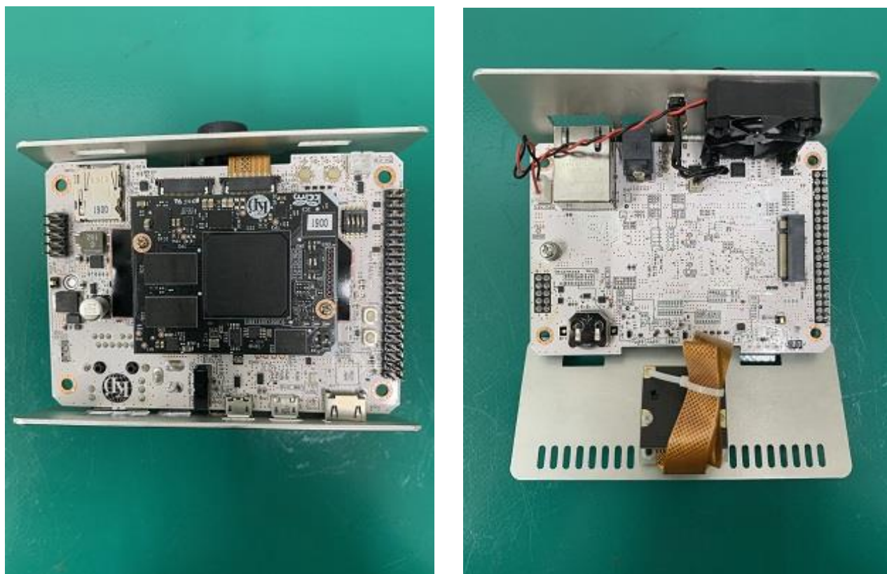
図 2-5 取り出した 前パネル、基板、後パネル
