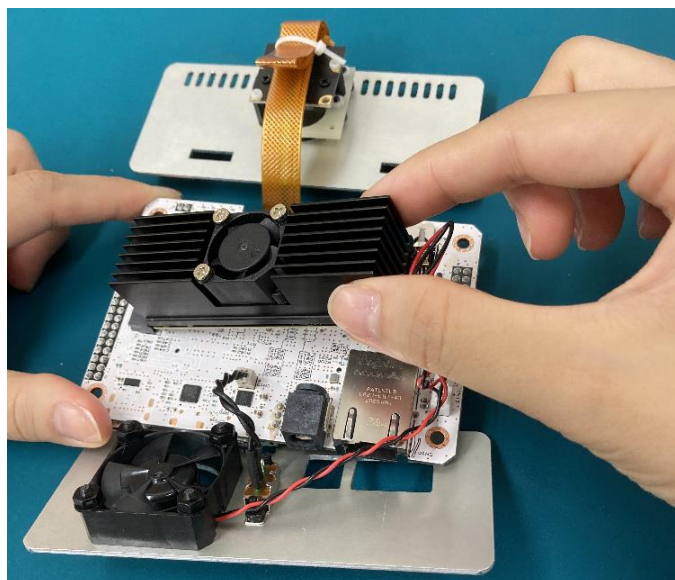
図 2-7 Mustang-M2BM-MX2 の挿入
