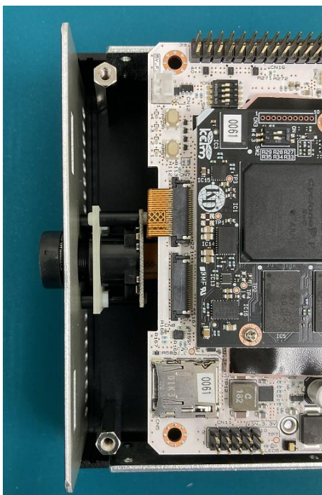
図 3-1 前パネルの装着
