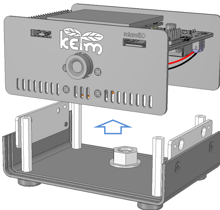
図 2-4 前後パネルと基板の取り出し
