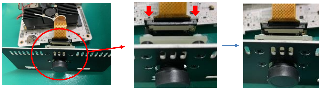
図 4-1 FPC の取り付け(カメラモジュール)
